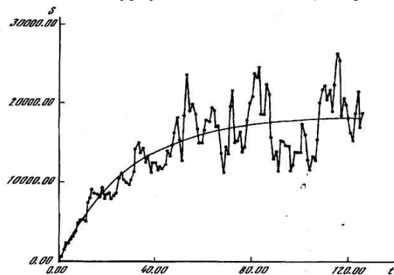
Рис. 11. Площадь территории России, млн. км 2 . Сравнение исторических данных с турбулентной моделью (построено автором)
