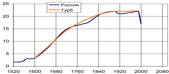
Рис. 11. Площадь территории России, млн. км 2 . Сравнение исторических данных с турбулентной моделью (построено автором)
