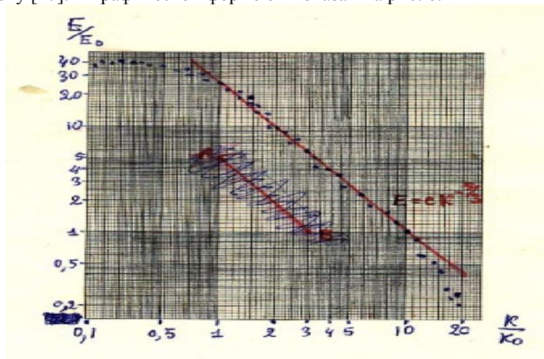
Рис. 6. Подобие спектров колебаний гидродинамических и финансовых (В) потоков, обнаруженное Колмогоровым (его авторский рисунок)
