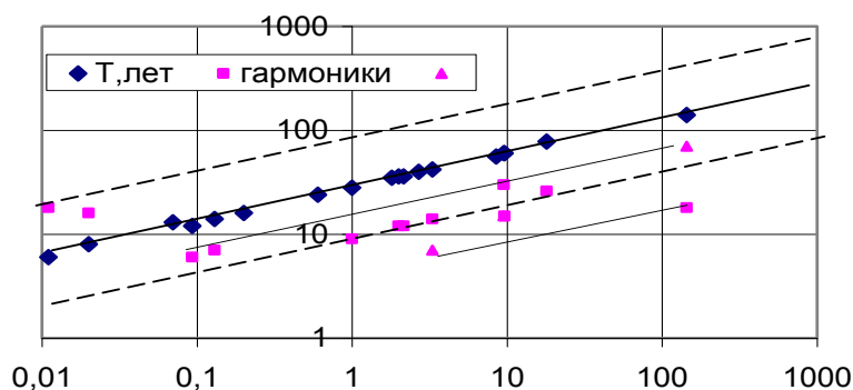
Рис. 8. Зависимость длины экономических волн различных государств от размеров их территории (сплошная линия — основная волна, штриховые — гармоники и обертоны). Сравнение с законом Колмогорова (прямые линии)
