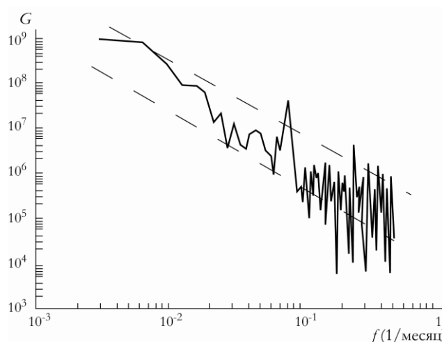
Рис. 7. Частотный спектр колебаний прироста населения, сопоставление статистических данных (кривая) с законом Колмогорова (штриховые линии)
