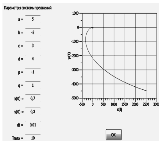
Рис. 3. Годограф скорости для системы уравнений (3) согласно модельной расчетной программе при значении свободного члена в первом уравнении p=-1
