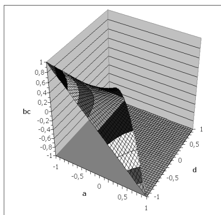
Рис. 1. Границы области устойчивости в трехмерном координатном пространстве a, d, bc
