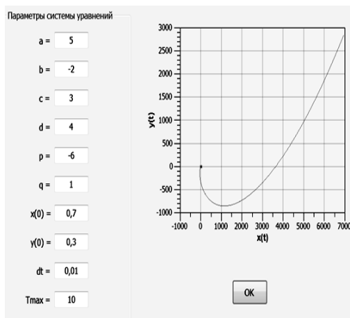
Рис. 2. Годограф скорости для системы уравнений (3) согласно модельной расчетной программе при значении свободного члена в первом уравнении p=-6
